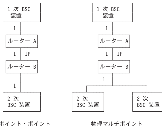
図 33. 物理 BSC リレー構成. 図の中の数字は、BSC リレーのグループ番号を表しています。
