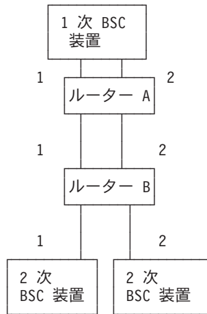
図34. バーチャル BSC リレー・マルチポイント構成. 図の中の数字は、BSC リレーのグループ番号を表しています。
