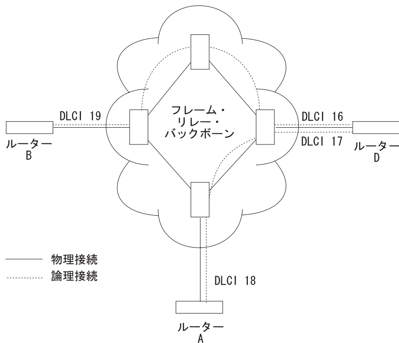
図21. FR ネットワーク内の DLCI
