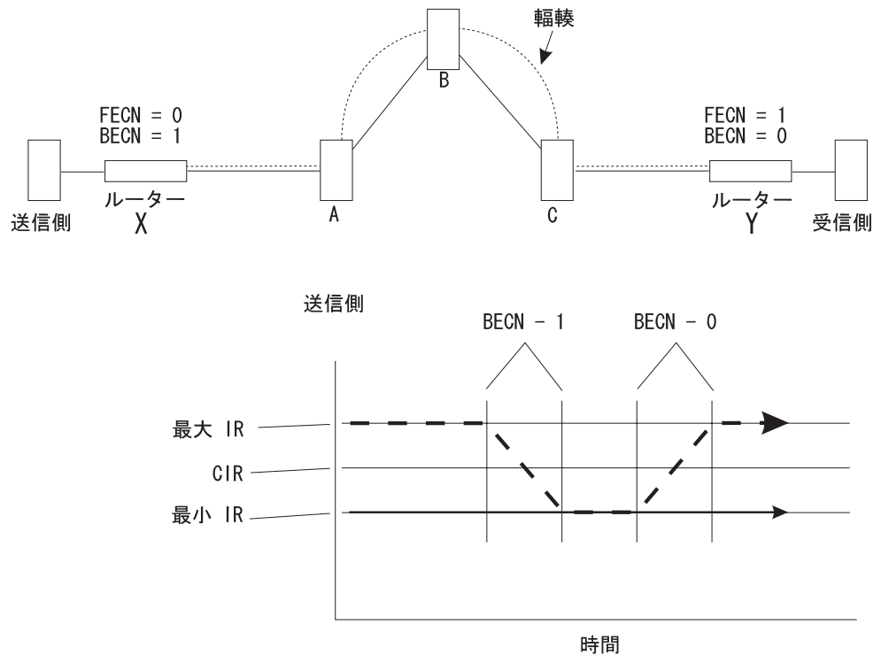
図 26. 輻輳通知と減速
