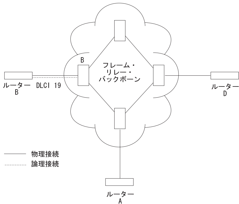
図23. フレーム・リレー・ネットワーク内の DLCI
