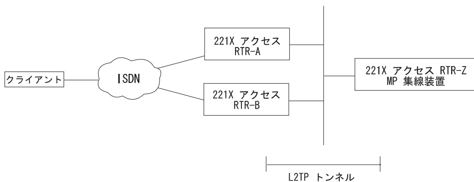
図 31. マルチシャシー MP
