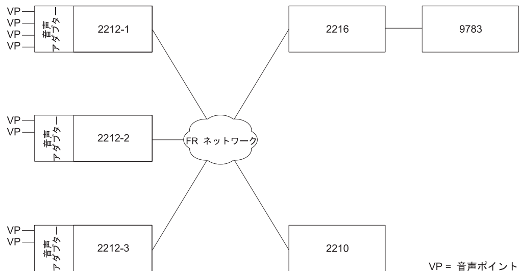
図 27. VoFR 構成のサンプル
