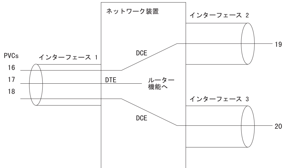
図 22. DTE および DCE 回線の多重化
